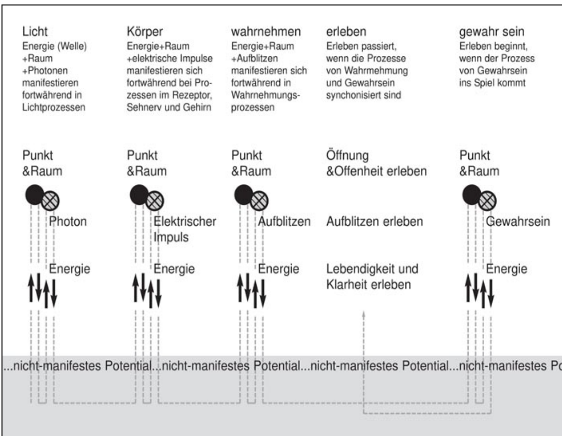
Bild 1 Quantenmodell mit 3Höfe-Prozessen
